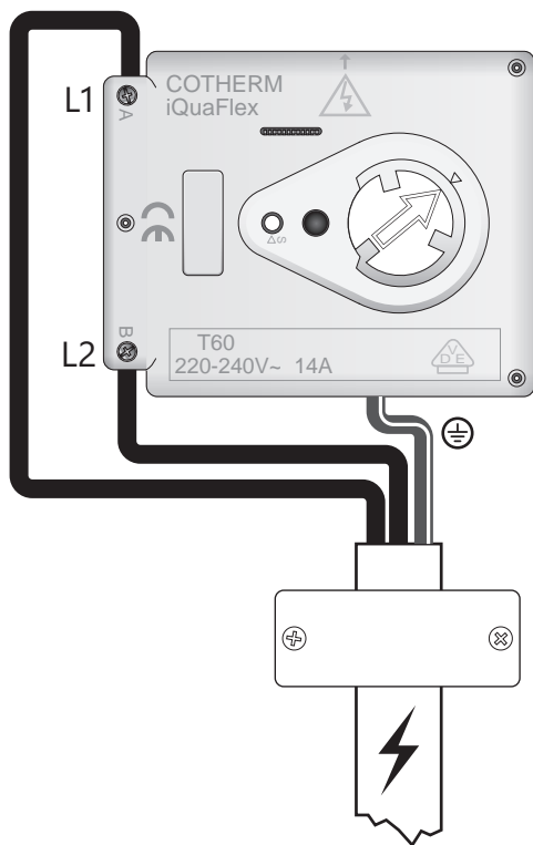
Электроподключение, схема
