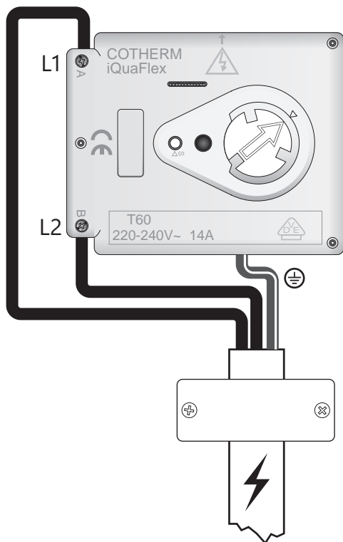
Schéma de câblage
